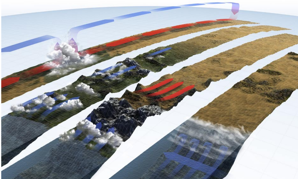
Die Wüsten-Grundtypen Schematische Darstellung der vier Arten von Wüste für GEO kompakt „Die Wüste“
