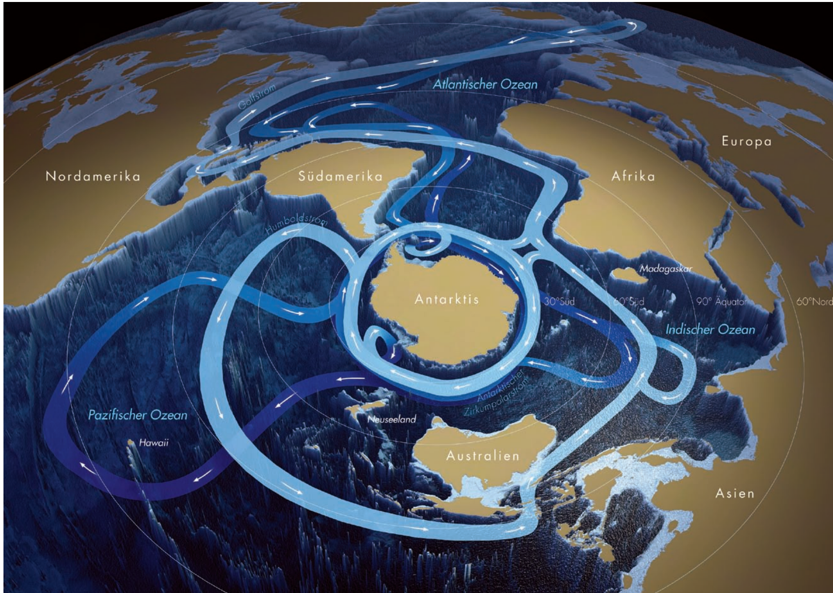
Das globale Förderband Darstellung des Wärmestroms für GEO kompakt „Wetter und Klima“
