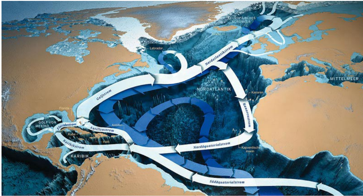
Das Strömungssystem im Nordatlantik Illustration über den Golfstrom für GEO kompakt „Wetter und Klima“
