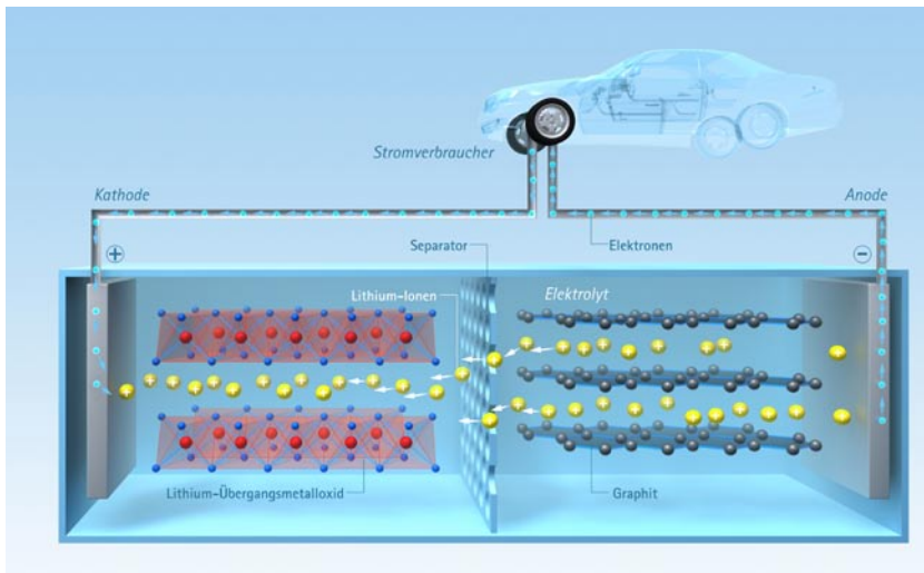
Lithiumionenakkumulator Illustration/Animation für Webauftritt von Merck
